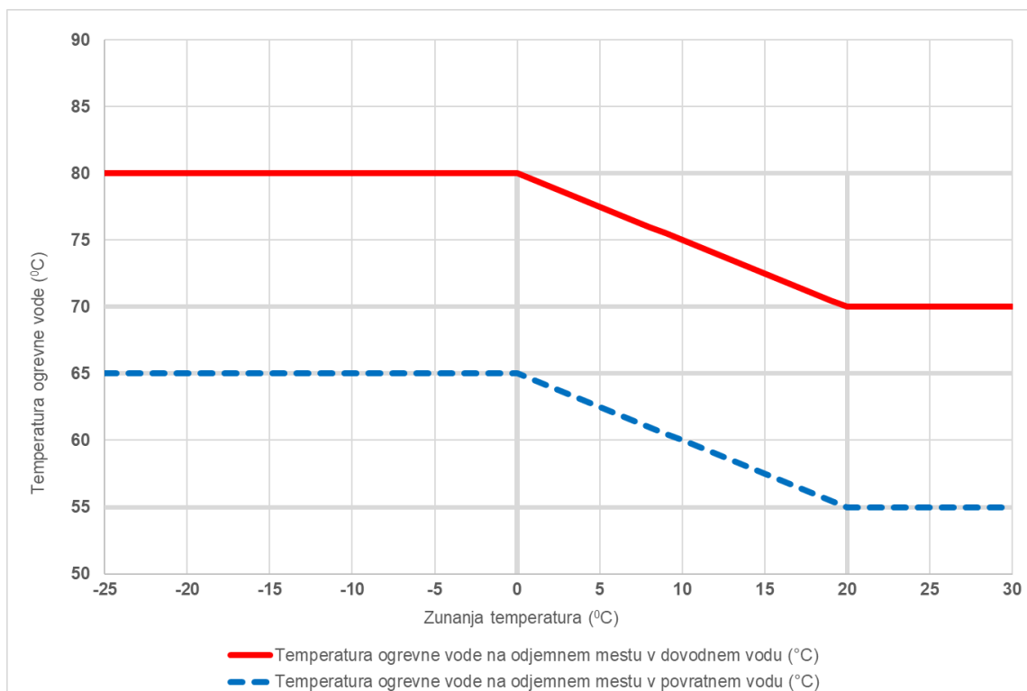
Diagram 4: Temperaturni diagram za zunanjo normno temperaturo -13 °C (2C toplovodni sistem 80/65 °C, NP 16)
