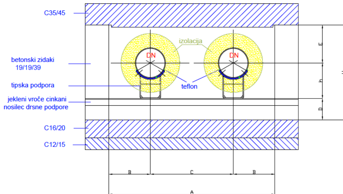
Slika 4: Detajl za izvedbo kinet na distribucijskem sistemu
