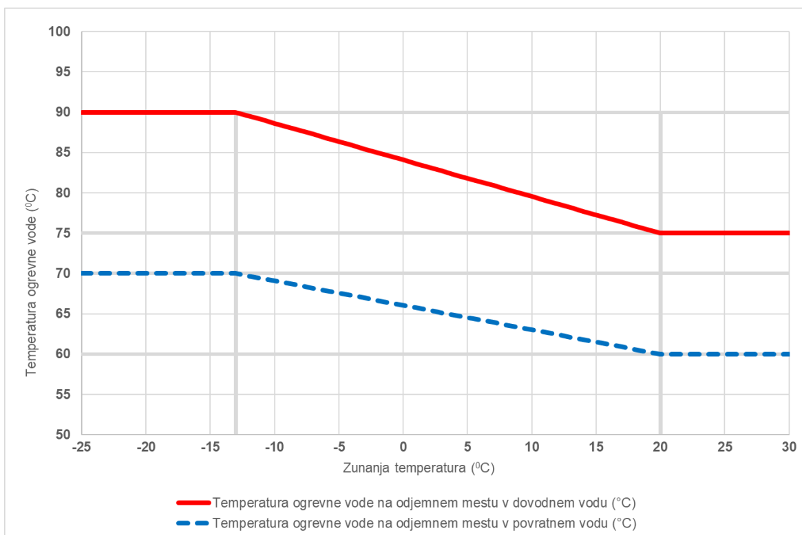
Diagram 3: Temperaturni diagram za zunanjo normno temperaturo -13 °C (2C toplovodni sistem 90/70 °C, NP 16 TPP 505, NP 6 CEP)
